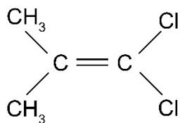
1,1 -dichloro-2,2-methylpropene
