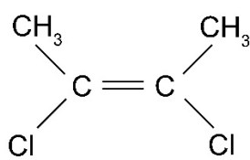
cis -2,3-dichlorobut
